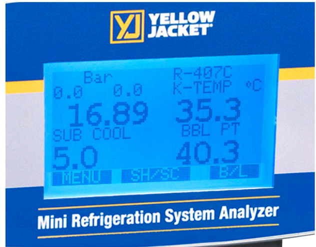
bar - Subcool
